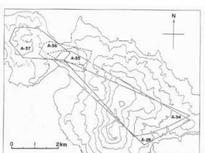
図13. 各雄（♂個体：A-25, A-34, A-35, A-36, A-37）の行動圏。 ——、成獣・亜成獣； - - - -、幼獣。
