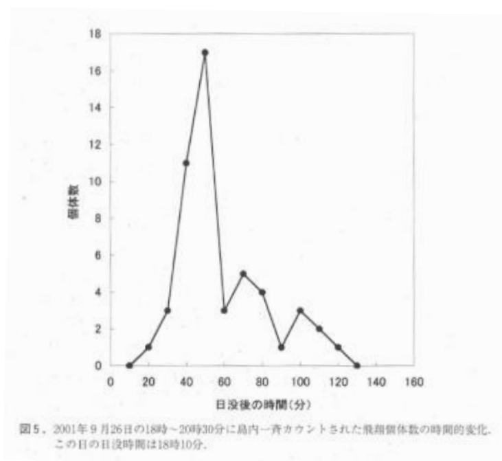
図 3-22 飛翔個体の時間的変化
